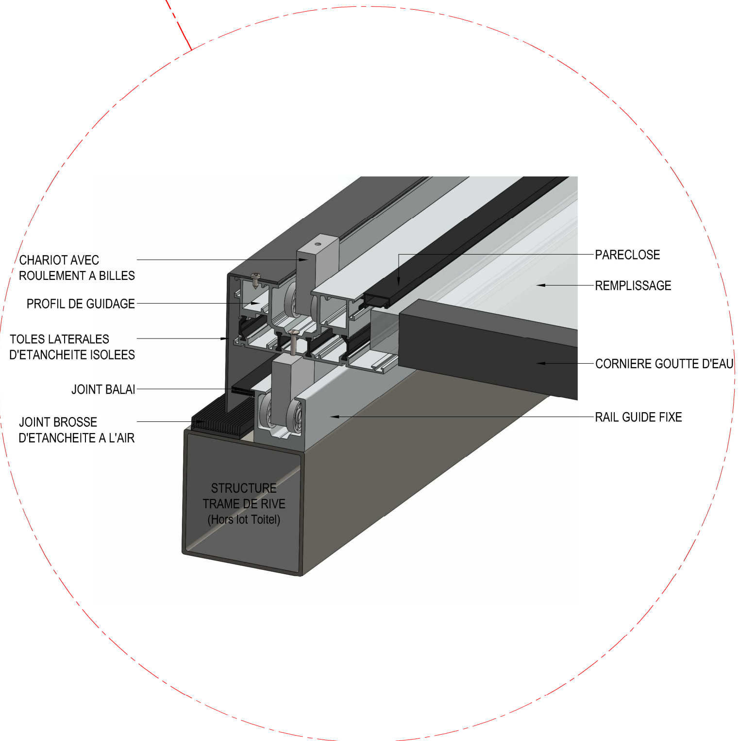
Coupes transversales sur toiture à 3 vantaux-Toiture ouverte
