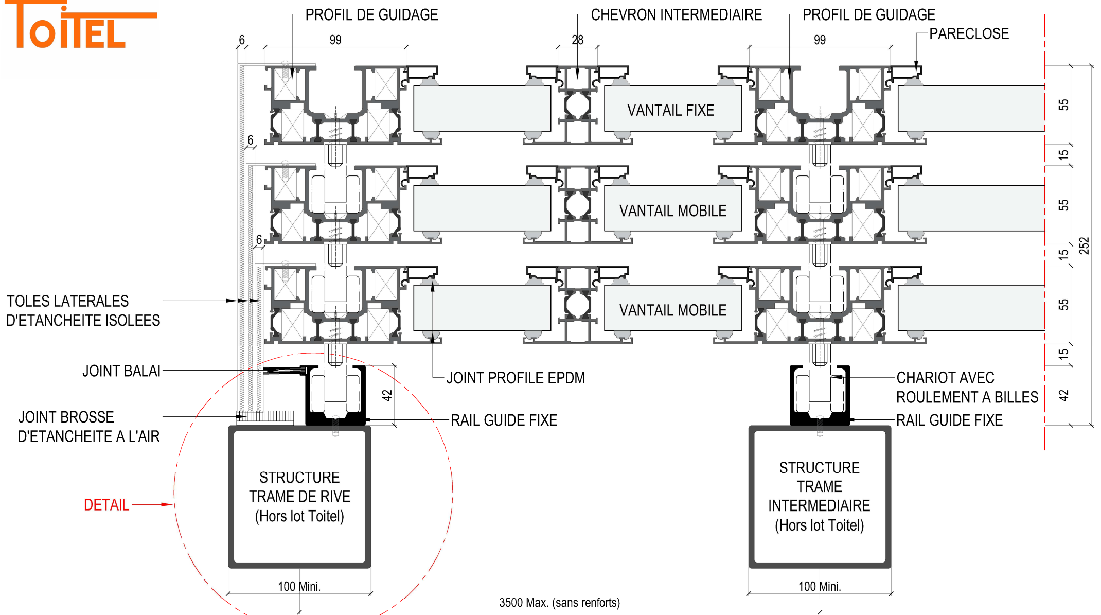
Coupes transversales sur toiture à 3 vantaux-Toiture ouverte
